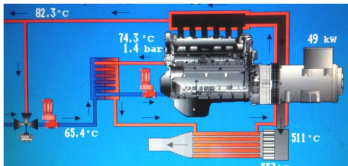
BHKW im Alters- und Pflegeheim: Prinzipschema
