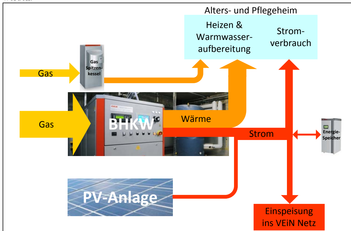
Prinzip des Energy-Hub im Alters- und Pflegeheim an der Lindenstrasse
