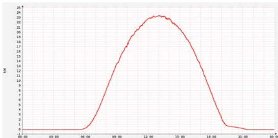
Wohnbaugenossenschaft Zähringer Einspeisung an schönem Sommertag
